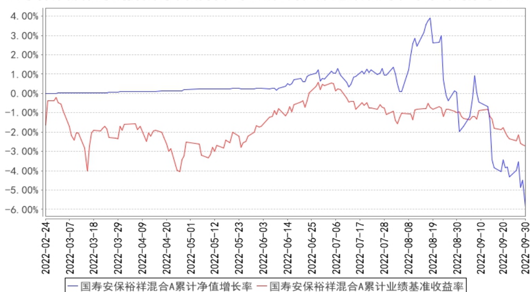
国寿安裕祥混合A累计净值增长率与同期业绩比较基准收益率的历史走势对比图
