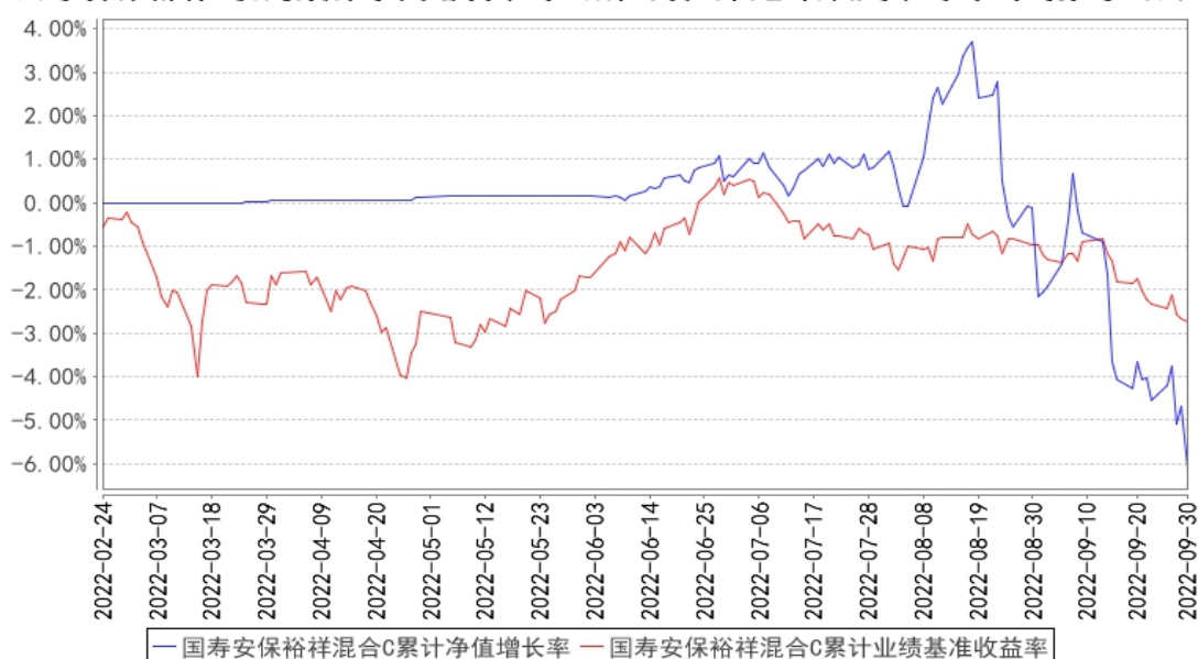
国寿安裕祥混合C累计净值增长率与同期业绩比较基准收益率的历史走势对比图
